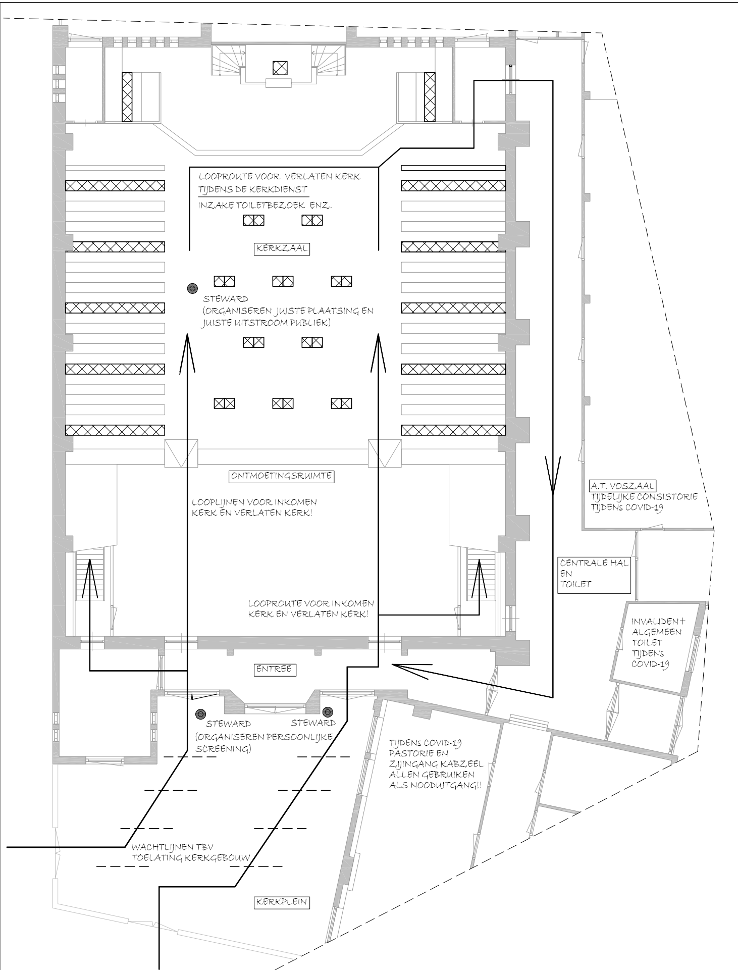
PLATTEGROND KERK DIJKSTRAAT 73 TE APPINGEDAM BEGANE GROND BEHORENDE BIJ GEBRUIKSPLAN COVID-19 VASTGESTELD DOOR KERKENRAAD D.D. 03-06-2020
